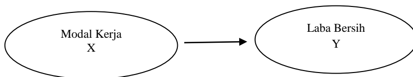
Gambar 1 Kerangka konseptual
