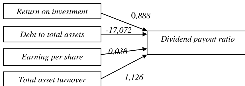
Gambar 2. Besarnya pengaruh masing-masing variabel independen terhadap variabel dependen
