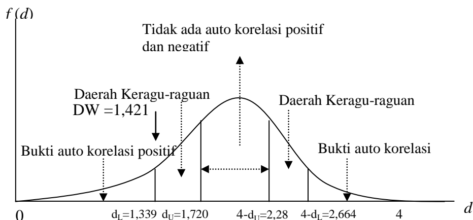
Gambar 1. Kurva Uji Statistik d Durbin-Watson
